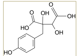
図1 ピシジン酸
